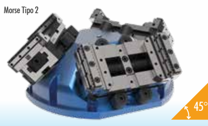
Morse Tipo 2
